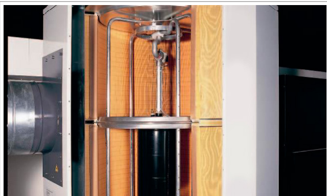
RoboCleanPlus filterreinigingssysteem dat zorgt voor automatische segmentsgewijze reiniging van de filterpatronen middels perslucht
